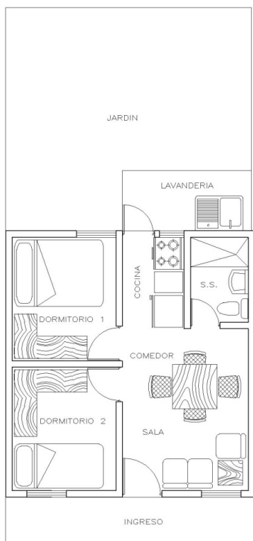
PLANTA ARQUITECTONICA
